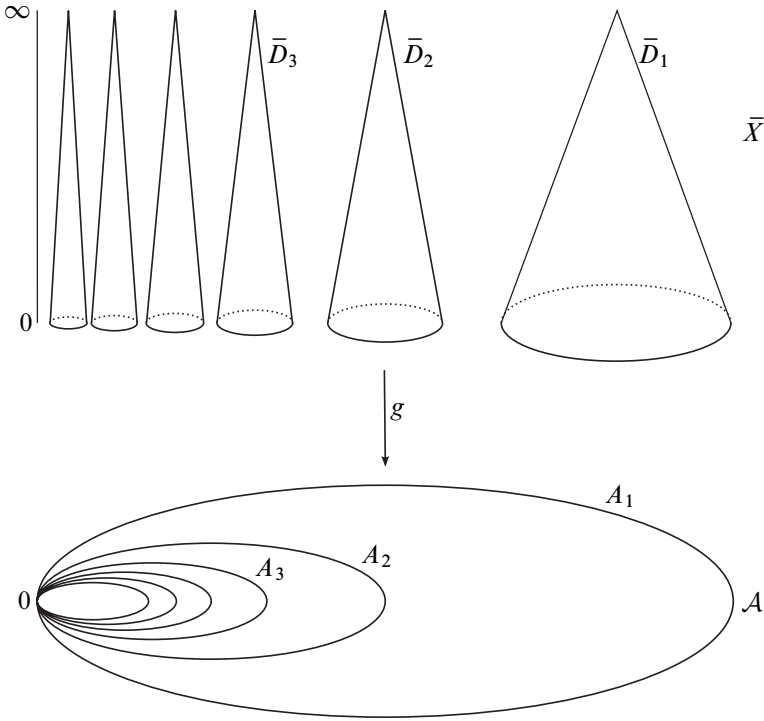
FIGURE 5: Le recollement \bar{X} \cup_g \mathcal{A} , homéomorphe à l'espace des sous-groupes fermés de \mathbb{R} \times \mathbb{Z}
