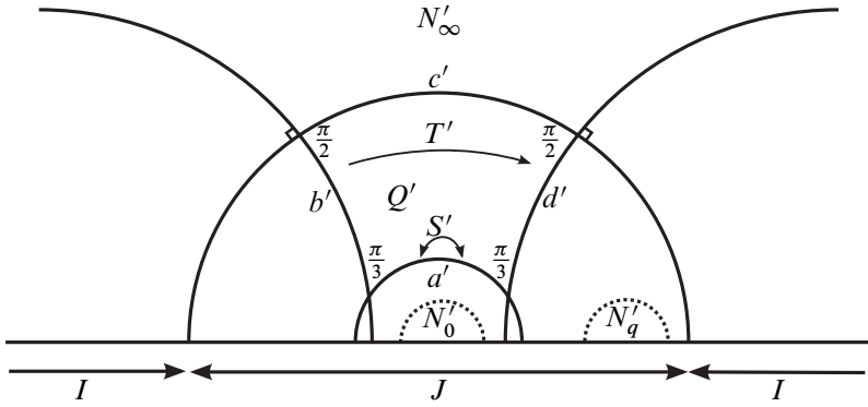
FIGURE 3: Le domaine fondamental Q' de l'orbifold E'
