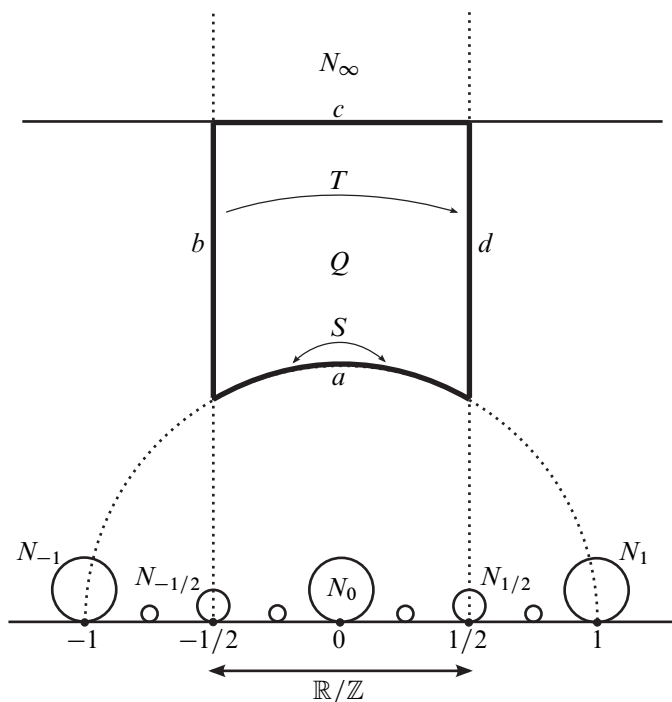
FIGURE 2: Le domaine fondamental Q de l'orbifold E
