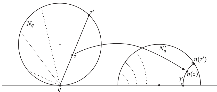
FIGURE 4: Le prolongement de l'homéomorphisme \eta de N_q sur N'_q
