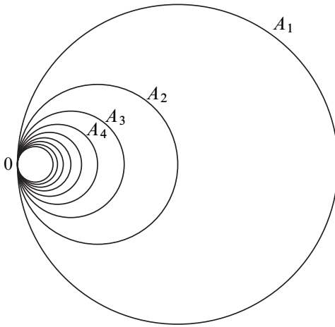
FIGURE 1: L'espace des "anneaux Hawaïens" \mathcal{A}
