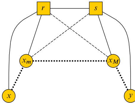
Figure 1. Lemma 2.8
