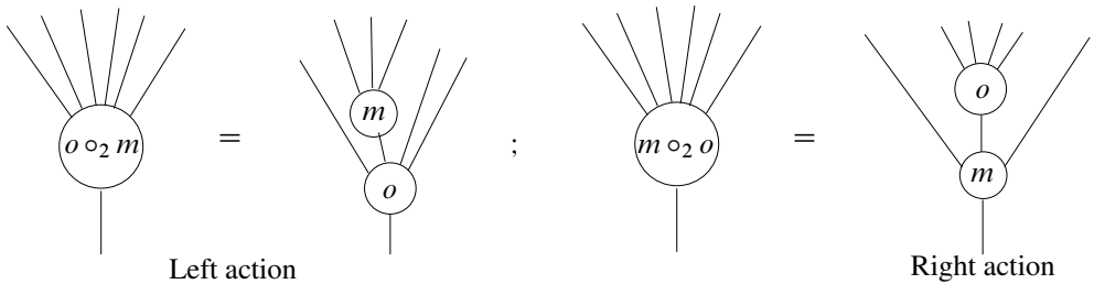
Figure 1: Infinitesimal action
