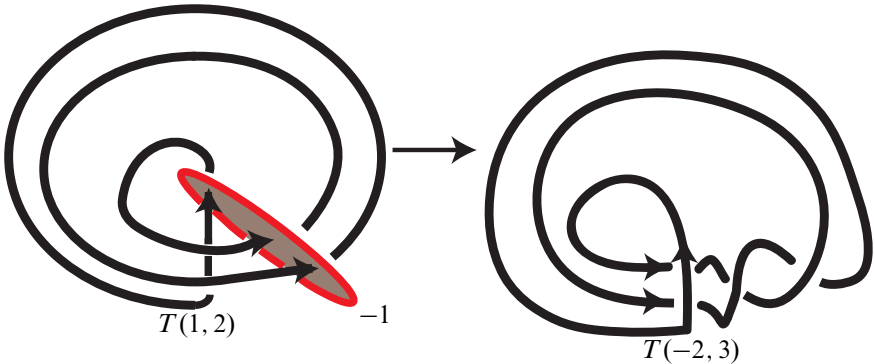
Figure 11: T(1, 2) \xrightarrow{(-1,3)} T(-2, 3)
