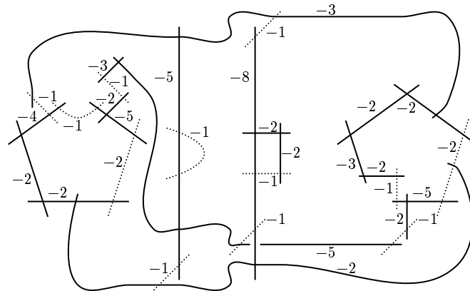
(d) Z = E(1) \# 16\overline{\mathbb{P}^2} . C_{3,1} : (-5, -2) . C_{3,1} : (-5, -2) . C_{16,11} : (-2, -2, -8, -2, -2, -2, -4) . C_{39,14} : (-3, -5, -5, -3, -2, -2, -3, -2) .
