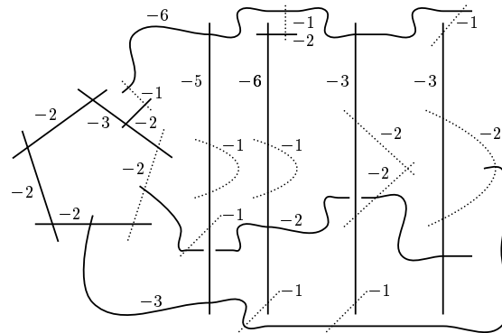
(d) Z = E(1) \# 10\overline{\mathbb{P}^2} . C_{7,4} = (-2, -6, -2, -3) . C_{48,17} = (-3, -6, -5, -3, -2, -2, -2, -3, -2) .
