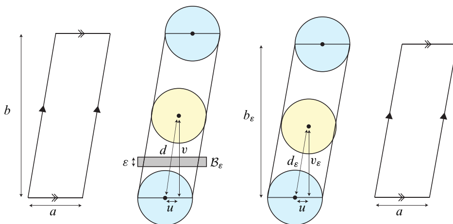
Figure 7: Chirurgie sur un tore plat
