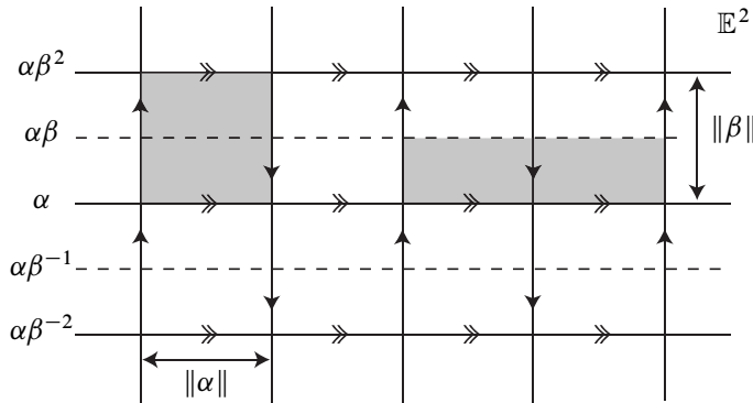
Figure 6: Revêtement universel de \mathbf{KI}
