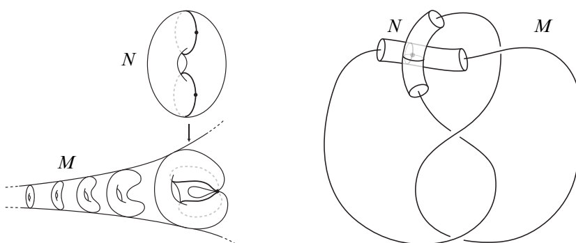
Figure 1: Fibre maximale (gauche) et nœud de huit (droite)
