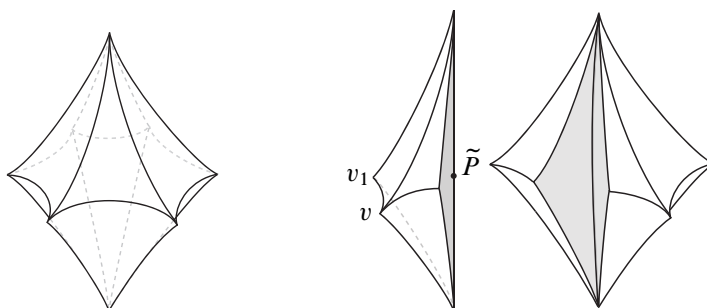
Figure 4: \mathcal{T} (gauche) et découpage de \mathcal{T} (droite)
