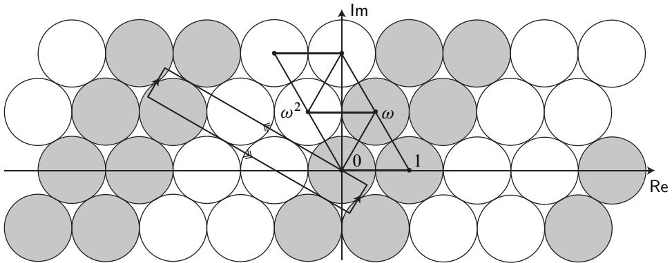
Figure 10: Empilement d'horoboules pour N1_1
